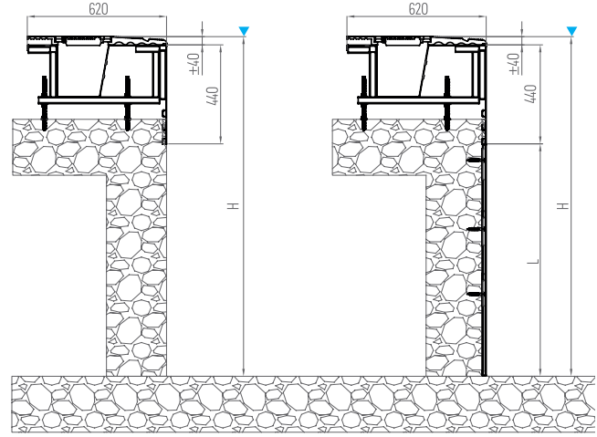
Seramik Taşma Kanalı
