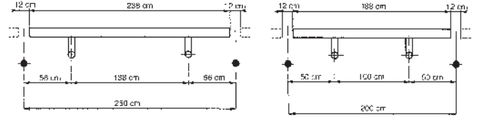
BRAKET SİSTEMİ «L» BOYU 500 MM' DEN AZ İSE.
