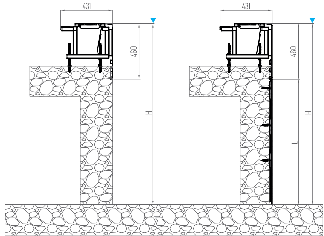
Taşma Kanalı (Seramiksiz)
