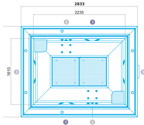
APOLO 6 Dikdörtgen Paslanmaz Çelik SPA + Lamba
